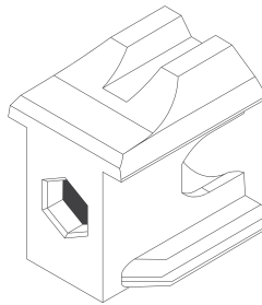
STRIKER
